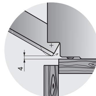
Detail Y
